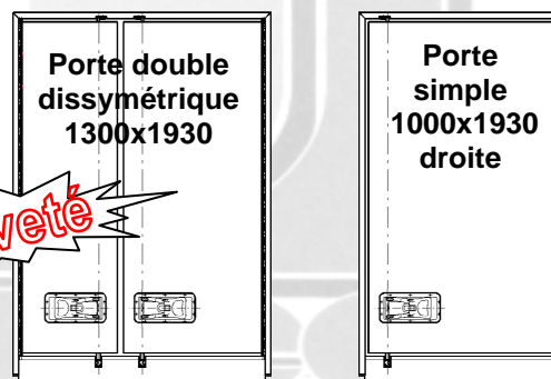
- AA - INCORPORATION HUISSERIE PORTE SIMPLE -
