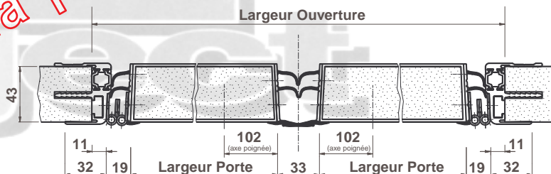
- INCORPORATION HUISSIERIE PORTE DOUBLE -
