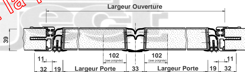
- INCORPORATION HUISSERIE PORTE DOUBLE -
