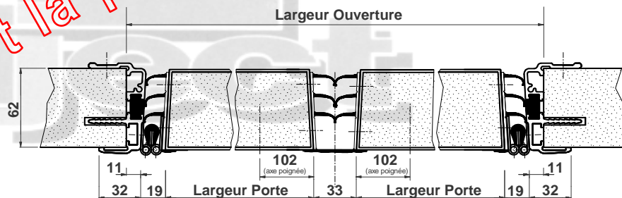
- INCORPORATION HUISSERIE PORTE DOUBLE -
