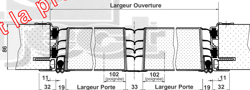
- INCORPORATION HUISSERIE PORTE DOUBLE -
